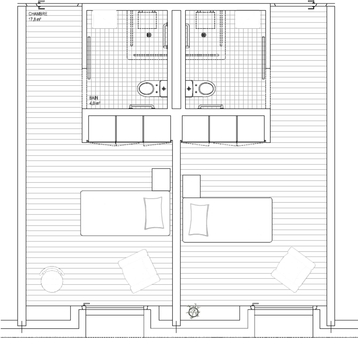
Schéma des chambres aux normes DAEMS
